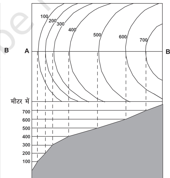
उत्तल ढाल
